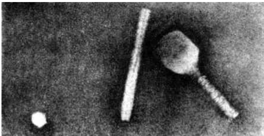
Рис. 6. Относительные размеры некоторых вирусов (электронная микрофотография с
