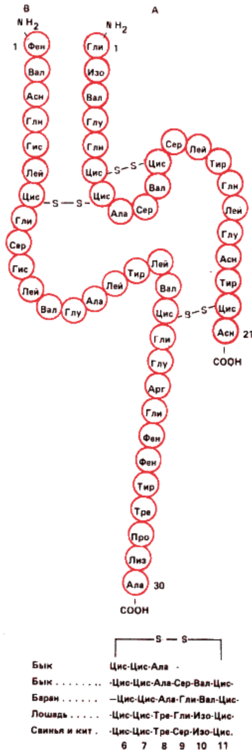
Рис. 3. На этом рисунке изображена схема молекулы инсулина. С сокращенными названиями, слагающих ее аминокислот мы познакомимся позже. Для нас сейчас важно другое: инсулин один из наименее специфичных белков (и это великое благо для страдающих диабетом; для их лечения можно применять инсулин крупного рогатого скота). Тем не менее почти каждый вид характеризуется некоторыми различиями в последовательностях. Так, в цепи А между шестым и одиннадцатым остатками цистеина, образующими дисульфидные мостики, последовательность аминокислот у быка, барана, лошади и свиньи неодинакова. Лишь у свиньи и кита она сходна, но они различаются по другим частям молекулы. Итак, специфичность
